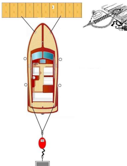
Bild 1: Korrekt förtöjning vid brygga/ponton
